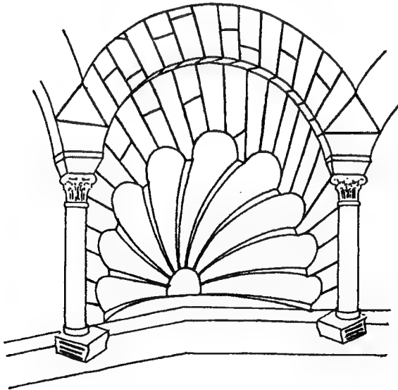
(شكل ٣٦) رسم لمقرنصة من مقرنصات أركان قبة المحراب ولمعد من العقود التي تمتطي المقرنصات
